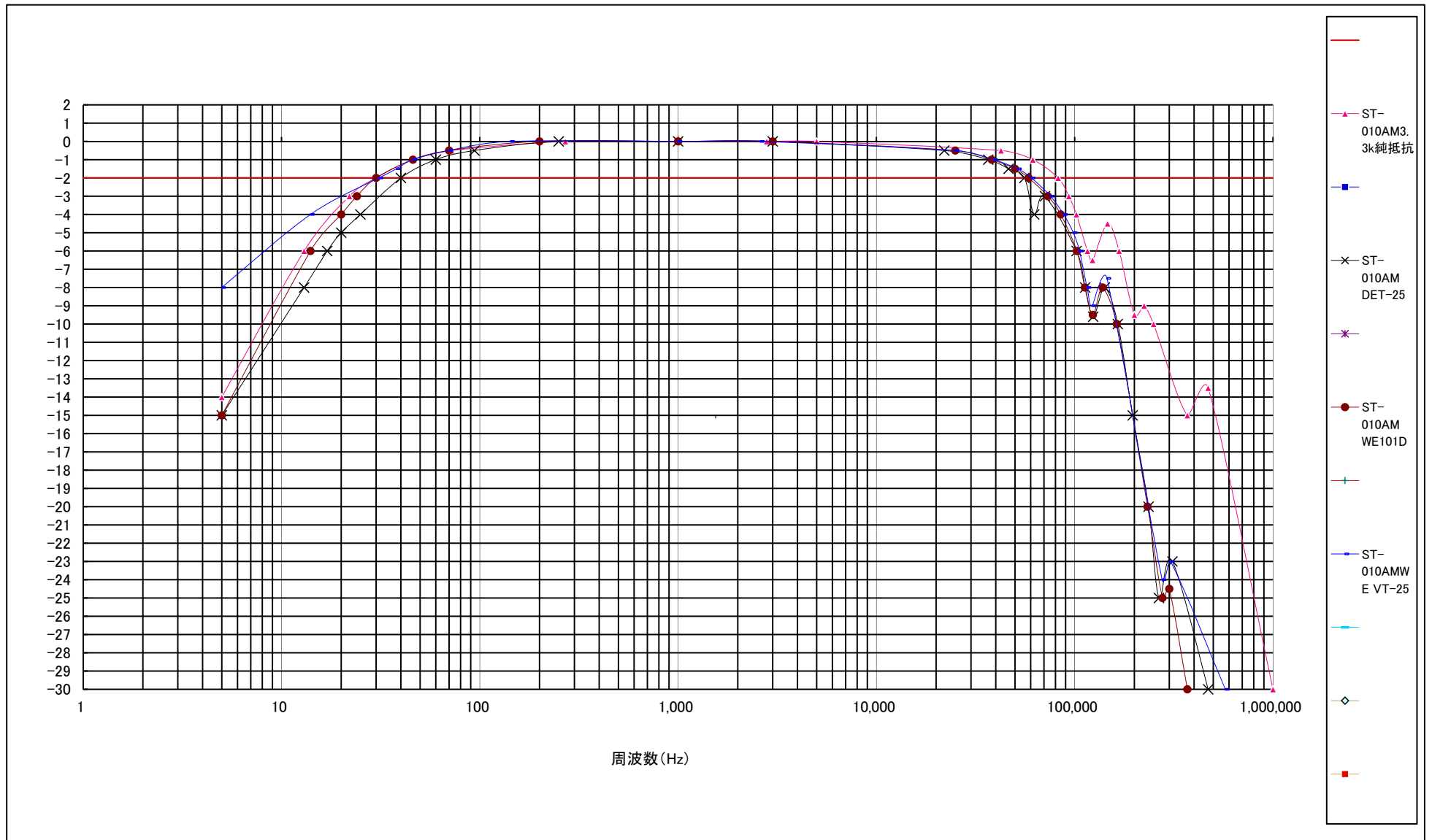
周波数特性
